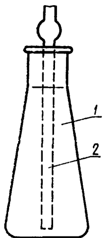
1 — приемник; 2 — барбатор
