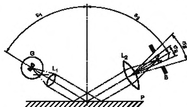
G — источник света; L_1 , L_2 — линзы; B — полевая диафрагма приемного устройства; P — лакокрасочное покрытие; \alpha_1 — угол падения, \alpha_2 — угол отражения ( \alpha_1 = \alpha_2 ); \sigma_0 — апертурный угол приемной системы; \sigma_s — апертурный угол изображения источника света; I — изображение источника света
