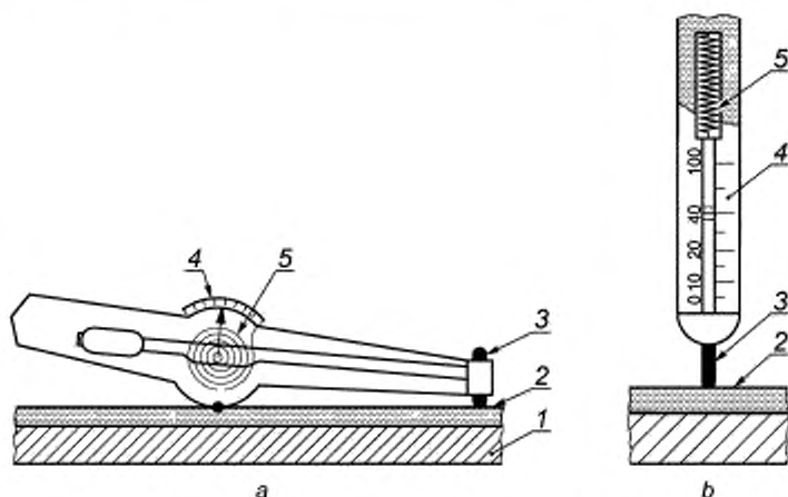
1 — окрашиваемая поверхность; 2 — покрытие; 3 — магнит; 4 — шкала; 5 — пружина
