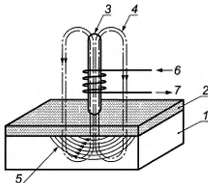
1 — окрашиваемая поверхность; 2 — покрытие; 3 — ферритный сердечник; 4 — переменное магнитное поле (ВЧ); 5 — вихревые токи; 6 — ток; 7 — сигнал измерения
