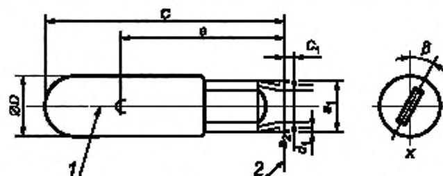
1 – базовая плоскость; 2 – базовая ось
