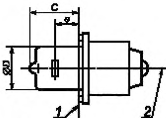
1 - базовая плоскость; 2 - базовая ось
