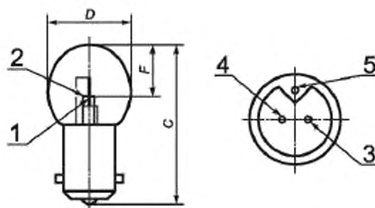
1 - основное тело накала; 2) - резервное тело накала; 3 - контакт основного тела накала; 4 - контакт резервного тела накала, 5 - контакт корпуса.
