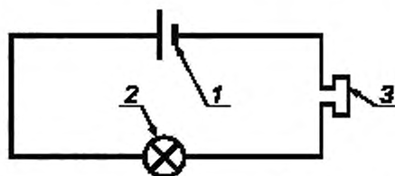
1 – источник постоянного тока напряжением 1 - 2,5 В; 2 – испытуемая лампа; 3 – головной телефон с сопротивлением 1600 - 2200 Ом
