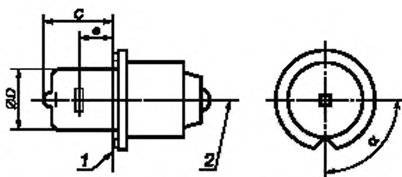
1 – базовая плоскость; 2 – базовая ось
