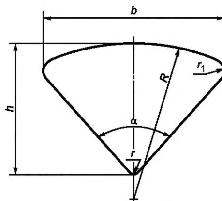
Рисунок А.2 — Конструкция секторных однопроволочных алюминиевых жил
