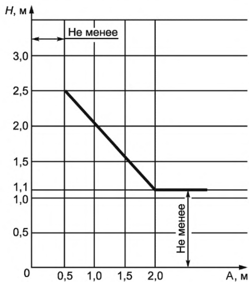
Рисунок 2 — Высота ограждения шахты в зависимости от расстояния от движущихся элементов лифта
