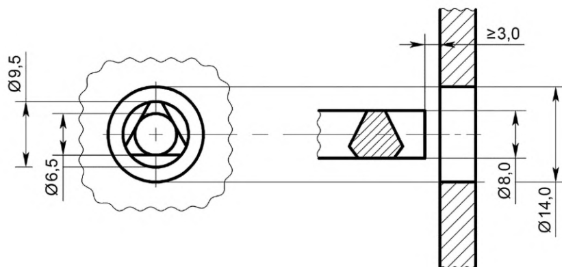
Рисунок Б.1 — Ключевина устройства отпирания замка
