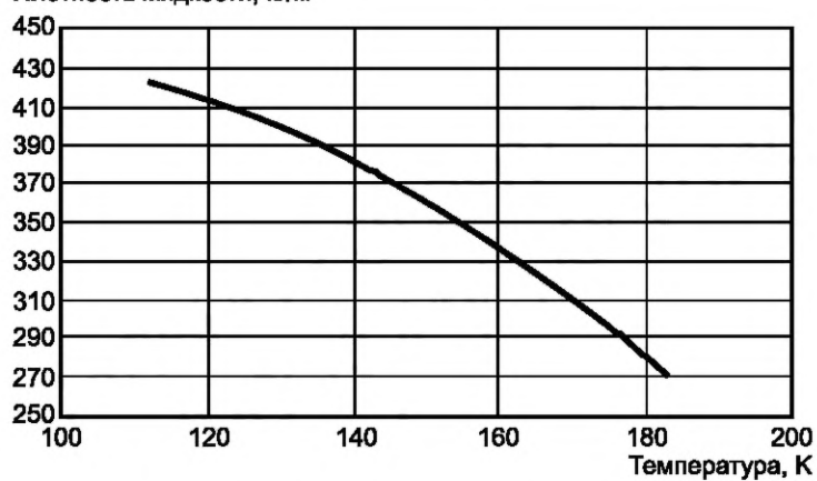
Рисунок А.2 — Плотность жидкого метана
