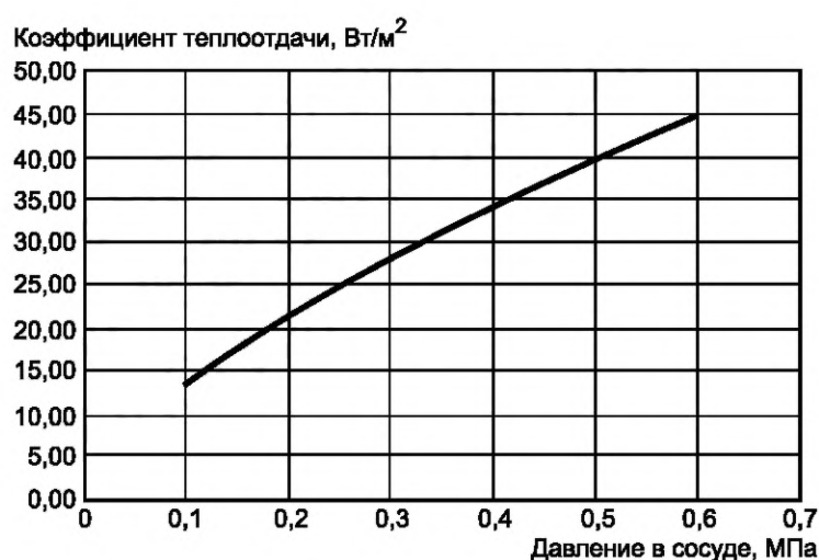
Рисунок Д.1 — Значения коэффициента теплоотдачи при естественной конвекции для метана
