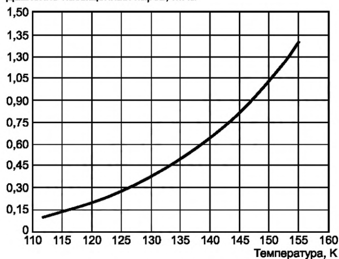
Рисунок А.1 — Равновесные температура и давление жидкого метана
