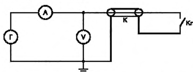
Г — генератор; А — амперметр; V — вольтметр; К — кабель; К п — ключ
