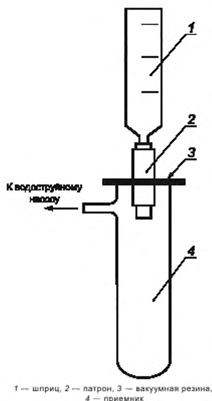
Рисунок Б.3 — Схема установки для проведения твердофазной экстракции
