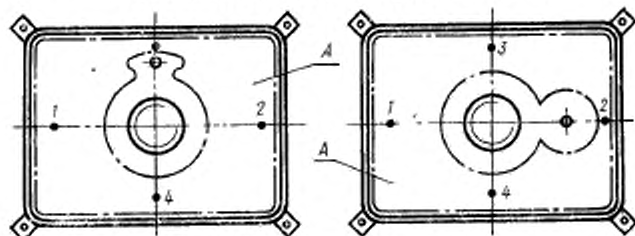
Вид на кинескоп со стороны горловины баллона
