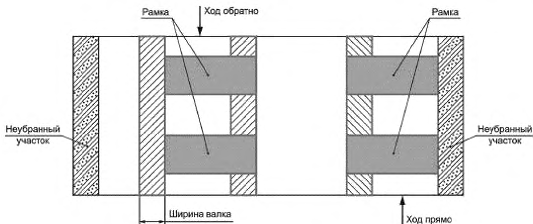
Рисунок 1 — Схема наложения рамок для учета потерь под валком и в межалковом пространстве
