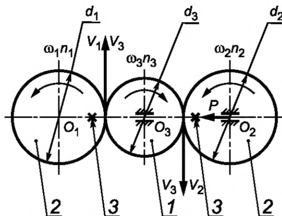
а) схема нагружения
