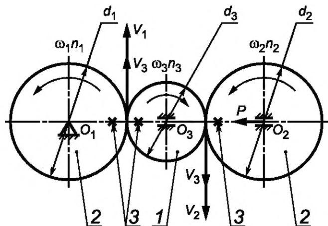
а) схема нагружения
