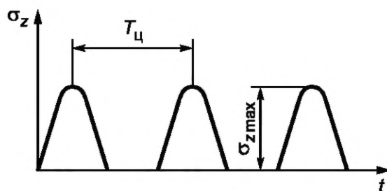
б) цикл напряжений
