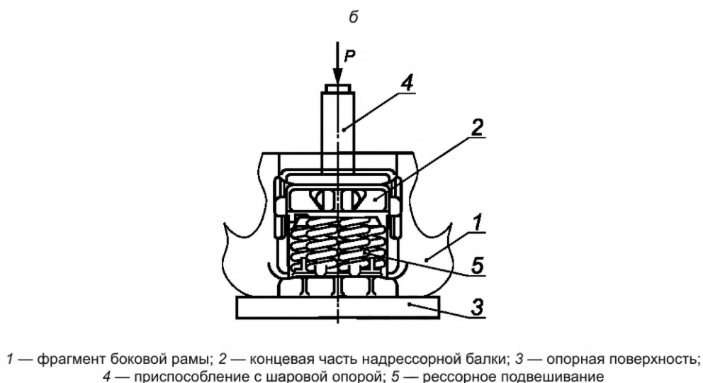
Рисунок 2 — Варианты схем установки и приложения силы к оснастке для испытаний клиньев
