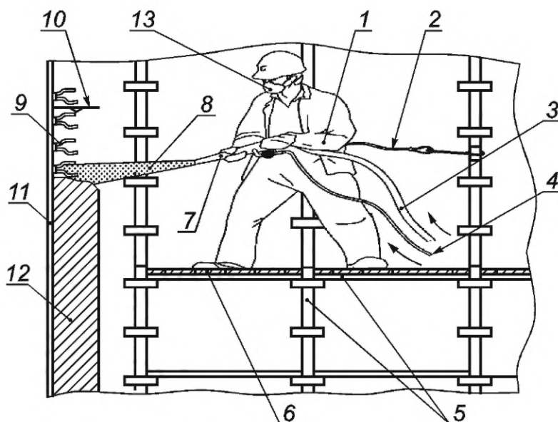
1 — торкретчик; 2 — фал предохранительного пояса; 3 — материальный (рабочий) шланг; 4 — шланг для подачи воды к соплу; 5 — инвентарные леса; 6 — сплошной дощатый настил; 7 — сопло торкретчика; 8 — факел с торкрет-массой; 9 — армирование футеровки (условно); 10 — ограничительный шаблон с выступом; 11 — корпус аппарата; 12 — футеровка; 13 — респиратор (СИЗ органов дыхания)
