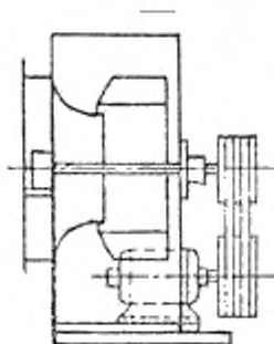
Рисунок 2 – Вентилятор с приводом
