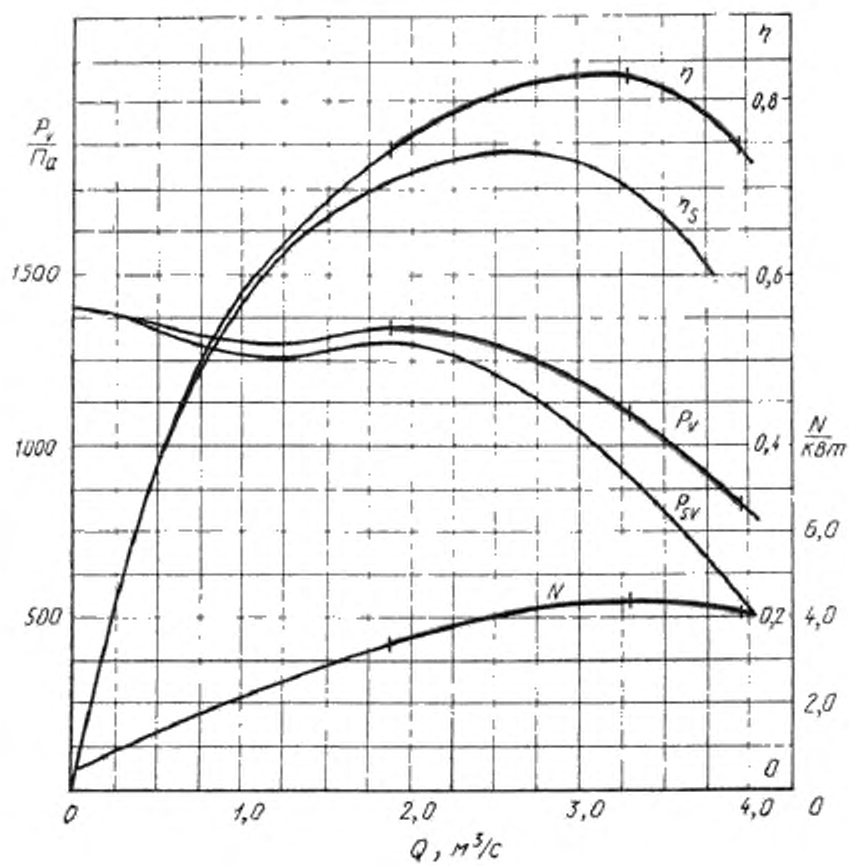
Рисунок Б 1 – Аэродинамическая характеристика вентилятора с выделенным рабочим участком
