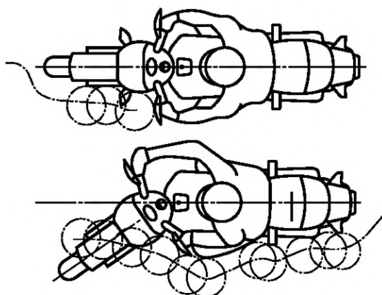
Рисунок 4 — Зоны обкатки испытательного устройства
