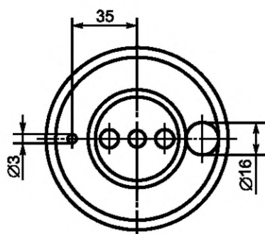
Рисунок 14 — Крышка формы
