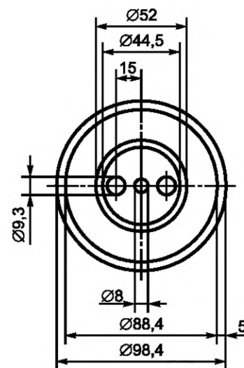
Рисунок 13 — Основание формы
