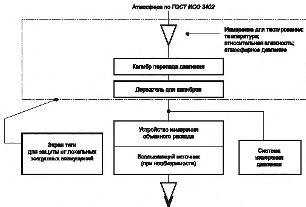
Рисунок А.2 — Типичное расположение калибровочного устройства
