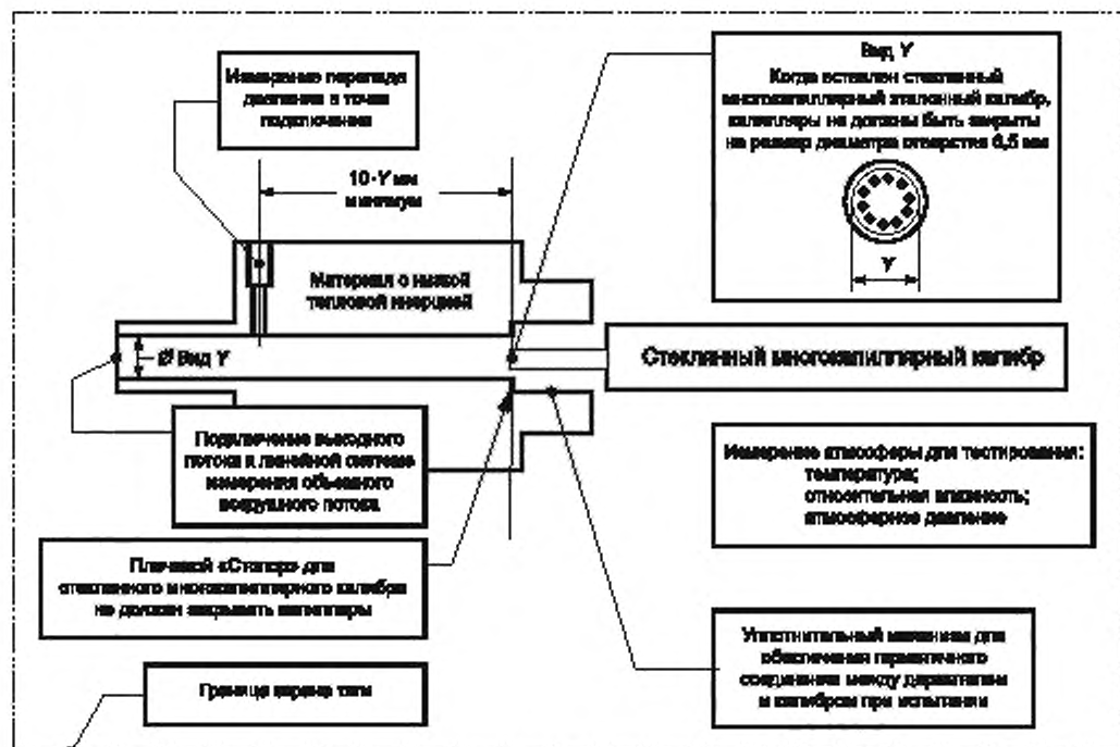
Рисунок А.1 — Основные свойства калибровочного устройства
