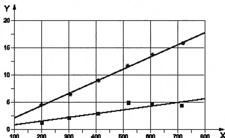
Рисунок В.2 — Взаимосвязь между r или R и m\Delta p (для фильтралочек)
