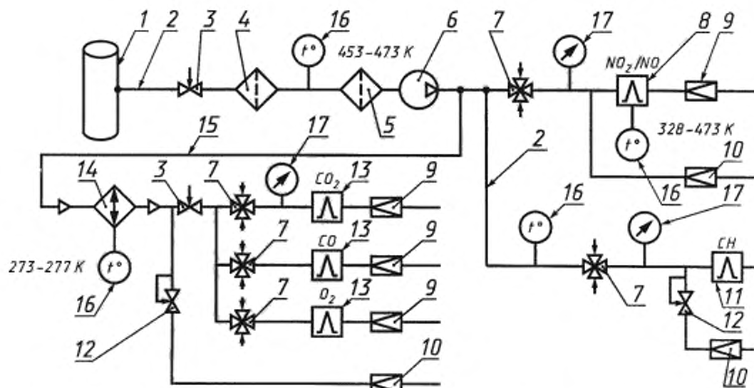
1 — пробоборборный зонд; 2 — нагретая линия отбора проб; 3 — регулирующий клапан; 4 — предварительный фильтр; 5 — фильтр; 6 — насос; 7 — система пробоборбора; 8 — пробоборборная магистраль с устройствами пробоборборки; 9 — селективный клапан для подвода поверочных газовых смесей; 10 — хемилуминесцентный газоанализатор; 11 — контроль потока через газоанализатор; 12 — контроль байпасного потока; 13 — газоанализатор пламенно-ионизационного типа; 14 — регулятор давления; 15 — газоанализатор недисперсионного типа с поглощением в инфракрасной области спектра; 16 — охладитель-конденсатор; 17 — линия отбора проб для анализа \text{CO} , \text{CO}_2 , \text{O}_2 ; 18 — термометр; 19 — манометр
