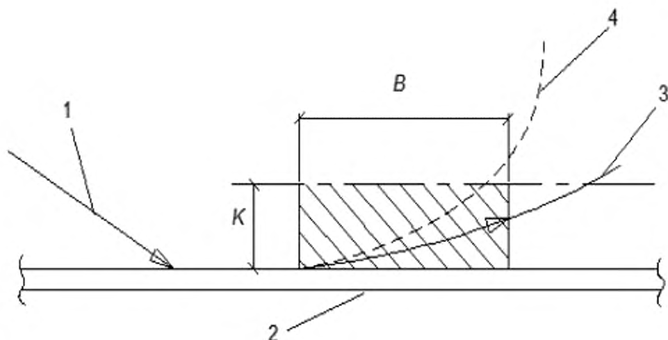
1 — траектория наезда; 2 — ограждение; 3 — траектория выбега, удовлетворяющая требованиям безопасности; 4 — траектория выбега, не удовлетворяющая требованиям безопасности
