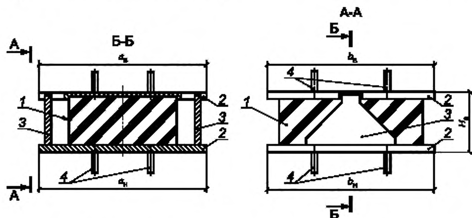
1 — резиновая опорная часть, 2 — закладные детали в пролетном строении и опоре; 3 — ограничители перемещения (упоры); 4 — анкера; a_n , a_n , b_n , b_n — размеры верхней и нижней закладных деталей в плане; H_c — высота опорной части с закладными деталями
