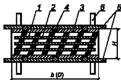
1 — резина; 2 — промежуточные стальные листы; 3 — утолщенные наружные стальные листы; 4 — стальные шпонки, 5 — закладные детали в пролетном строении и опоре, 6 — анкера; b(D) — размеры опорной части в плане, H — высота опорной части
