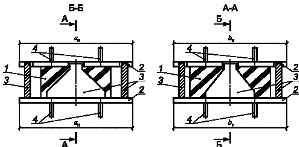
1 — резиновая опорная часть; 2 — закладные детали в пролетном строении и опоре; 3 — ограничители перемещения (упоры); 4 — анкера; a_B , a_N , b_B , b_N — размеры верхней и нижней закладных деталей в плане; H_0 — высота опорной части с закладными деталями
