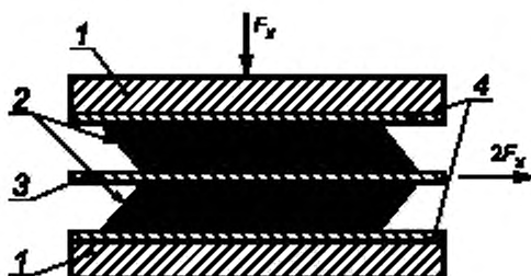
1 — плиты пресса; 2 — образец для испытаний; 3 — подвижная плита; 4 — выравнивающие плиты с пазами, предназначенными для предотвращения проскальзывания резиновой опорной части; F_x — поперечная сила
