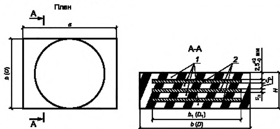
1 — резина; 2 — промежуточные стальные листы; a , b(D) — размеры опорной части в плане; b_1(D_1) — размеры в плане стальных листов; b_2 — толщины стальных листов; b_2 — толщины промежуточных слоев резины; H — высота опорной части
