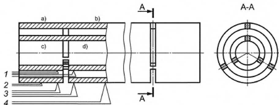
а) — охранный торцевой участок испытательной трубы; б) — зона измерения испытательной трубы; с) — охранный торцевой участок нагревательной трубы; д) — зона измерения нагревательной трубы
