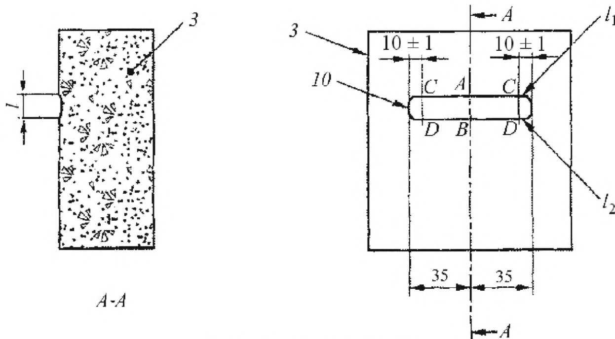
Рисунок В.4 – Схема измерения канавки
