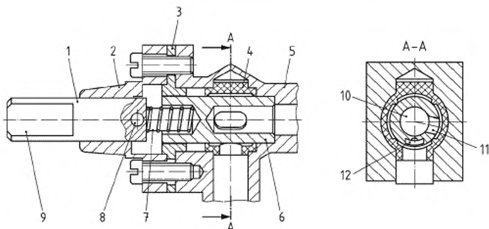
1 – рабочий шпindel; 2 – крышка; 3 – вставка; 4 – уплотнение пробки; 5 – корпус; 6 – пробка; 7 – пружина; 8 – стопорный штифт; 9 – плоские грани для ручки; 10 – выходное отверстие; 11 – основной поток газа; 12 – уменьшенный поток газа
