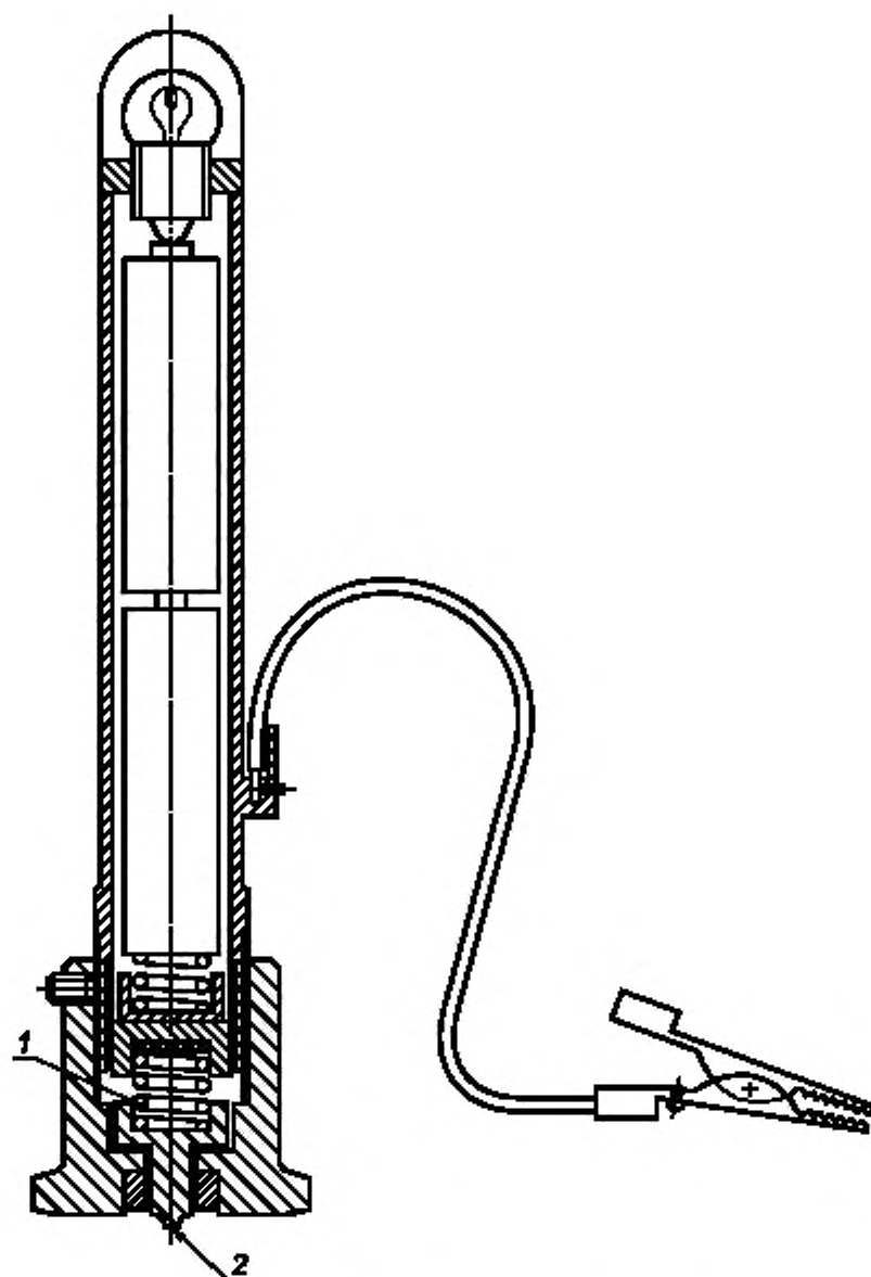
1 — пружина с усилием нагрузки 10 Н; 2 — наконечник, которым проводят испытание царапанием (стальной шарик диаметром 1 мм)
