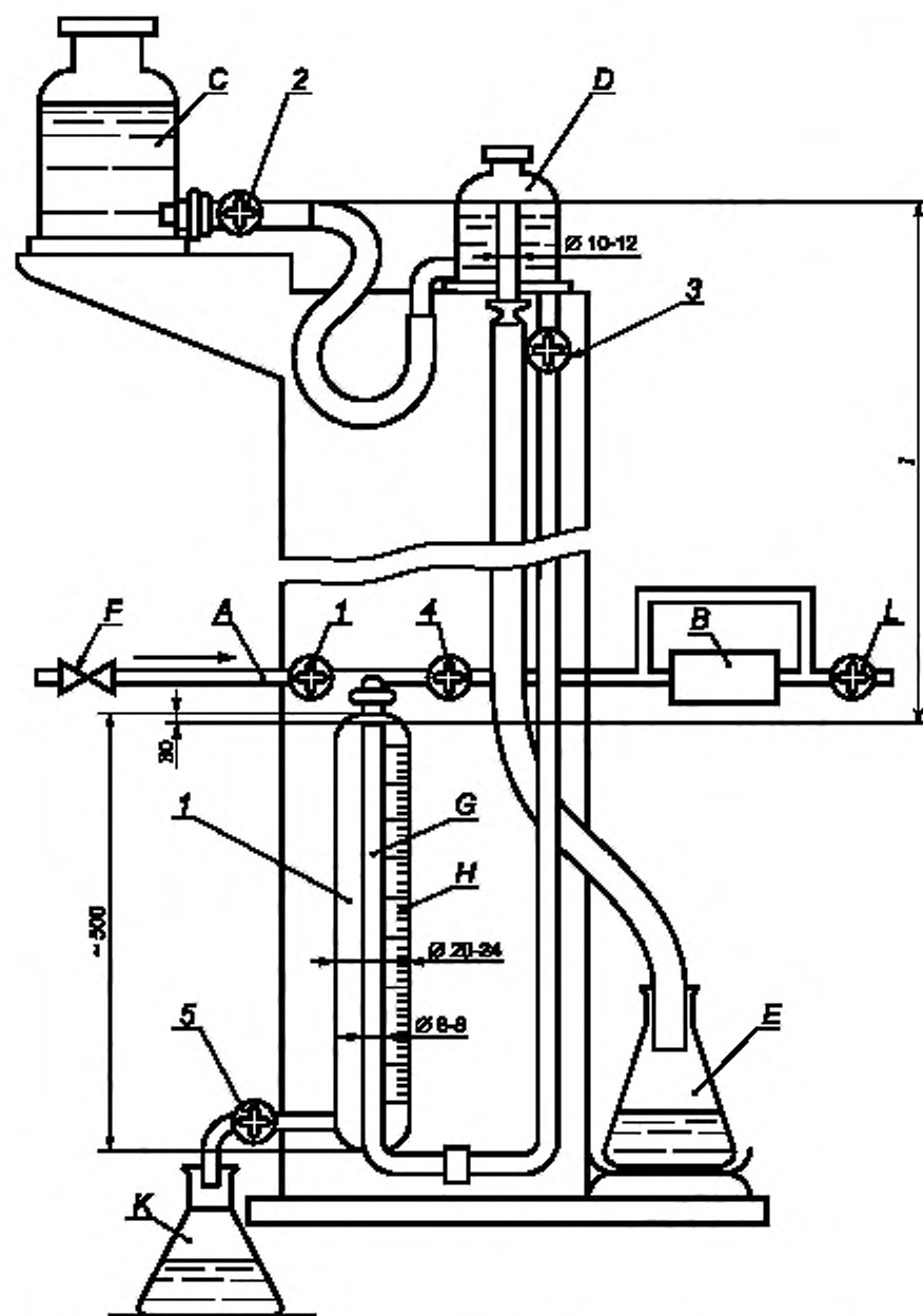
l — расстояние между уровнем воды в сосуде линии изгиба трубки; А — вход; В — испытуемый образец; С — емкость с водой; D — сосуд с постоянным уровнем воды; E, K — переливные сосуды; F — регулятор; G — трубка; H — измерительная бюретка; L — выход клапана; 1—5 — ручные краны
