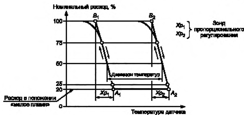
а) Терморегулятор непрерывного действия
