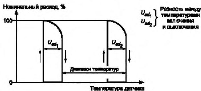
б) Двухпозиционный терморегулятор
