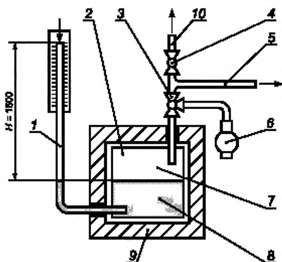
1 — трубка со шкалой, мм; 2 — теплоизолированный сосуд под давлением; 3 — трехходовой кран; 4 — кран; 5 — патрубок для присоединения испытуемого образца; 6 — компрессор; 7 — воздушная камера объемом 1 дм 3 ; 8 — вода; 9 — теплоизоляция; 10 — напорная трубка
