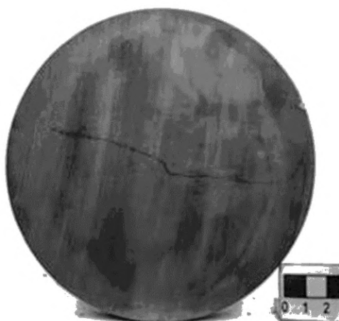
a — внешний вид (холодный рез)
