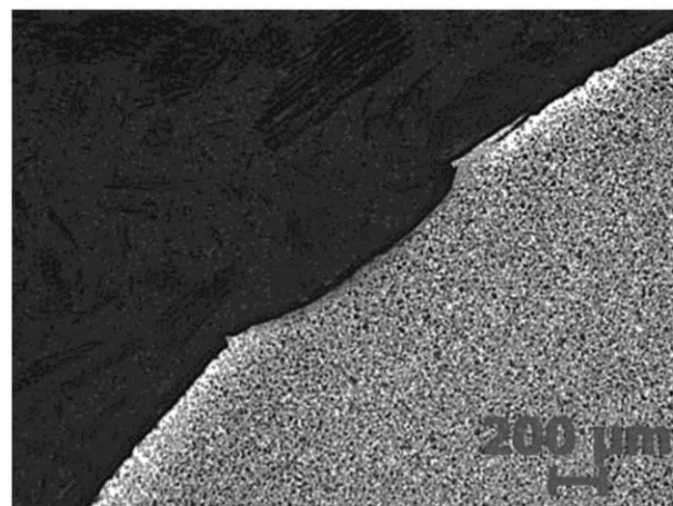
б — микроструктура после травления в 4 %-ном растворе азотной кислоты в спирте, 50 x
