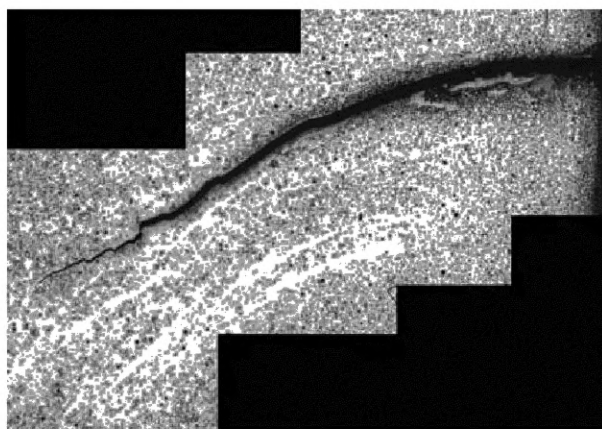
е — вид дефекта в поперечном сечении микрошлифа после травления в реактиве Обергоффера, 50 х
