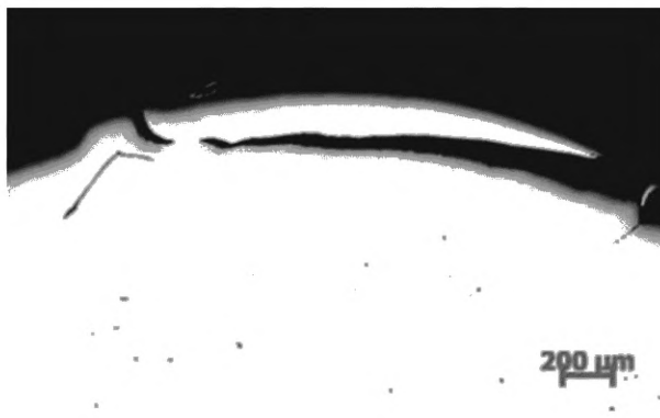
з — вид на полированном микрошлифе 50 х
