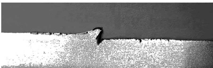
Рисунок Б.57 — Заусенец (внешний вид) (термин 3.4.4)
