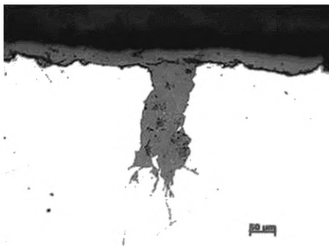
б — вид дефекта на микрошлифе до травления, 100 ×
