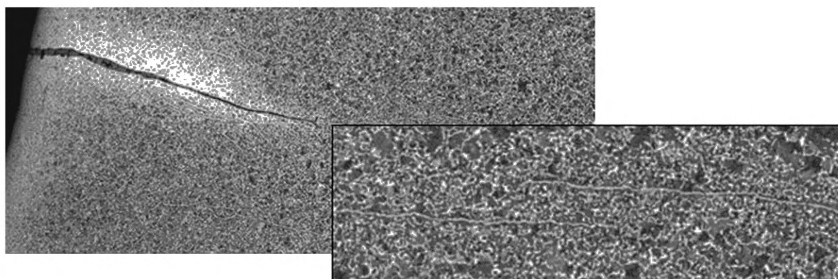
д — вид дефекта в поперечном сечении микрошлифа после травления в реактиве Nital, 50 х
