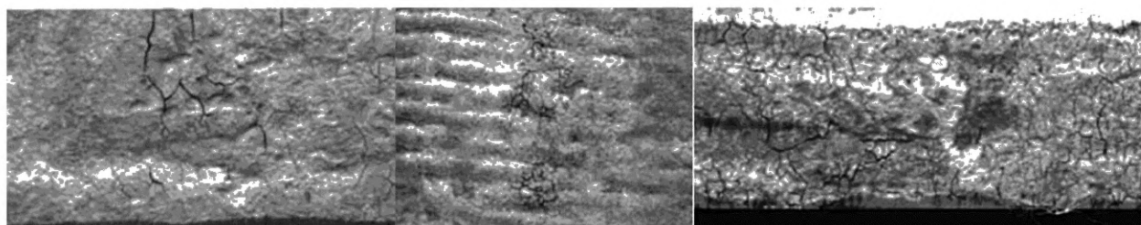
в — сетчатые трещины на поверхности непрерывного слитка (горбушка) после удаления окислы травлением в горячем 50 %-ном растворе соляной кислоты
