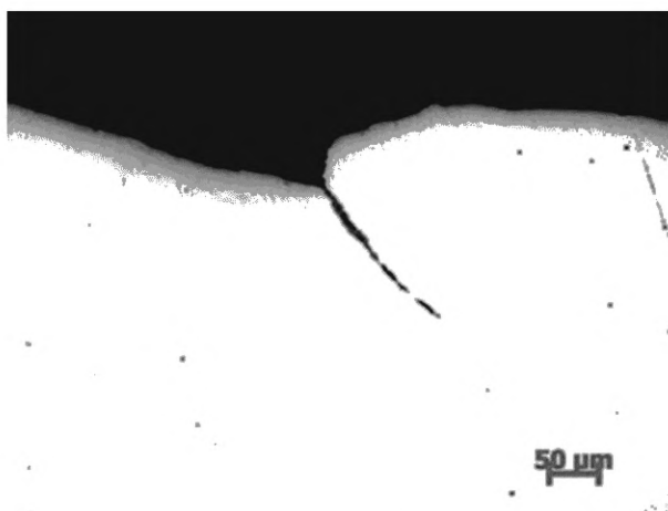
а — вид дефекта на микрошлифе до травления, 100 х
