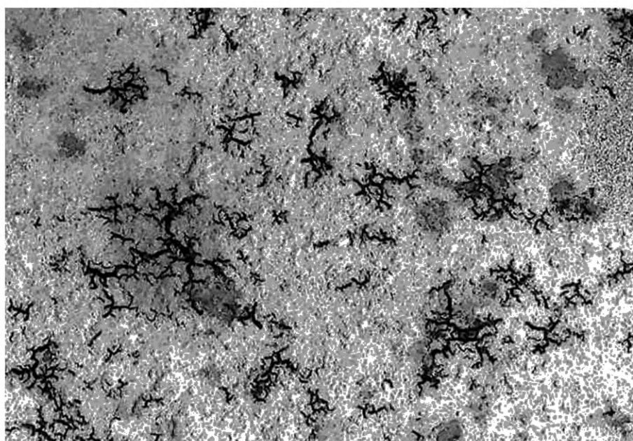
г — внешний вид паучообразных трещин после удаления окислы травлением
