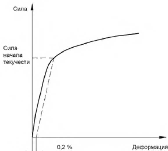
Рисунок 2 — Определение силы начала текучести
