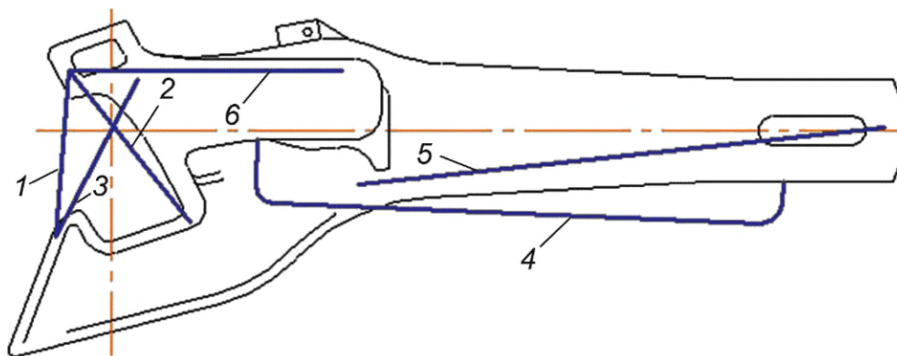
1—6 — скобы
