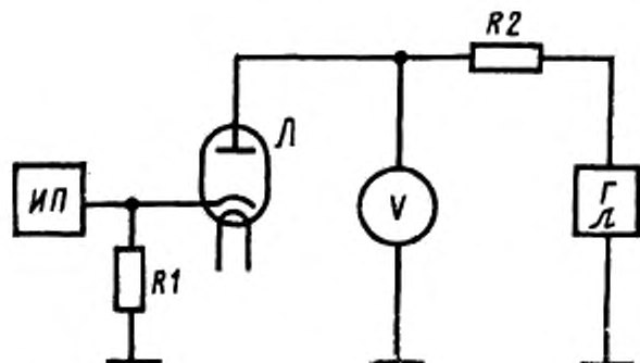
Л — испытываемая лампа; ИП — импульсный вольтметр или осциллограф; R1 — безындуктивный измерительный резистор; R2 — безындуктивный ограничительный резистор; V — импульсный вольтметр; Г — генератор импульсов.
