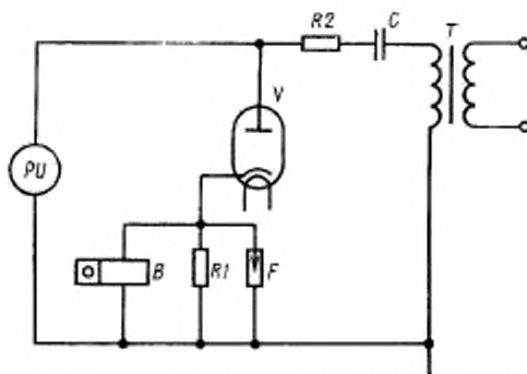
T — высоковольтный трансформатор; C — конденсатор; R1 — измерительный безындуктивный резистор; R2 — ограни- тельный безындуктивный резистор; PU — импульсный кило- вольтметр (допускается применение вольтметра для косвенного контроля обратного напряжения анода); B — счетчик искрений; F — разрядник; V — испытываемая лампа
