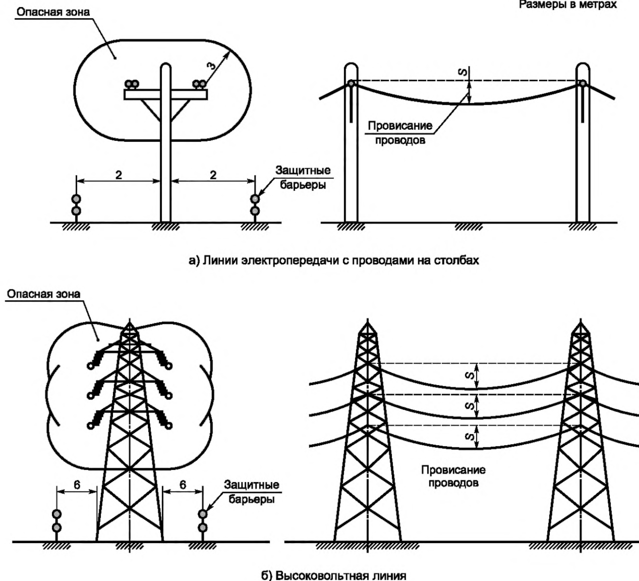
Рисунок 1 — Зазоры от токонесущих проводов линии электропередачи
