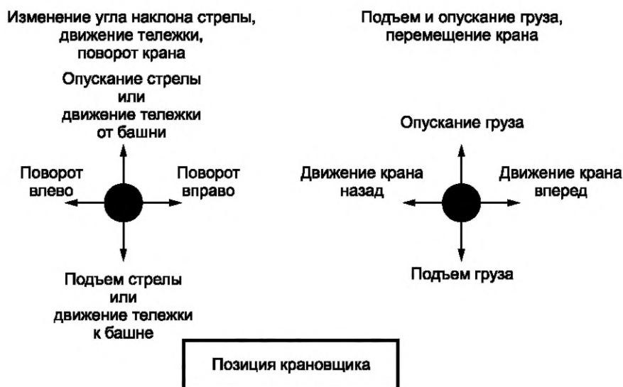
Рисунок 1 — Схема расположения основных органов управления башенным краном
