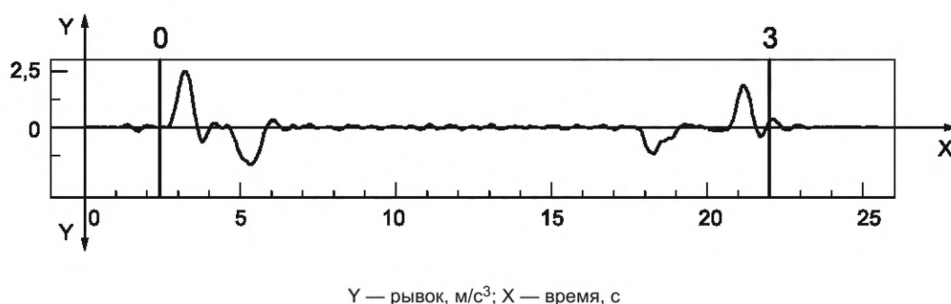
Рисунок 4 — Сигнал рывка
