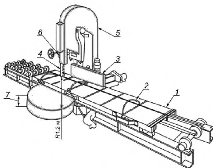
1 — подвижный стол; 2 — зажимное устройство; 3 — направляющая (базирующая) линейка; 4 — полотно ленточной пилы; 5 — разъемное защитное устройство для шкива ленточной пилы; 6 — передвижное разъемное защитное устройство для полотна ленточной пилы; 7 — низ подвижного стола на высоте не более чем 100 мм
