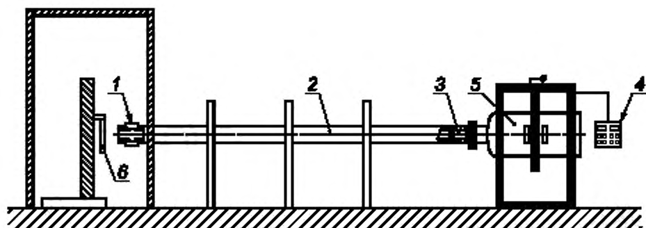
1 — измеритель скорости снаряда; 2 — ствол; 3 — перемещаемый снаряд; 4 — пульт управления; 5 — баллон сжатого воздуха; 6 — испытуемый объект
