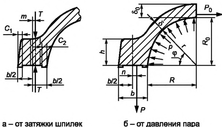
Рисунок 10.1 — Силы, действующие на фланец корпуса цилиндра
