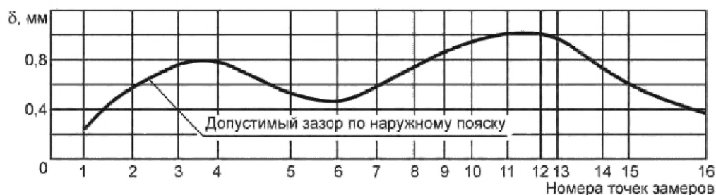
Расчет перемещений деталей проточной части при затяжке корпуса ЦВД
