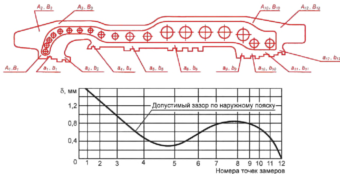
Схема измерения зазоров в горизонтальном разрезе корпуса ЦВД Расчет перемещений деталей проточной части при затяжке корпуса ЦВД Исходные данные
