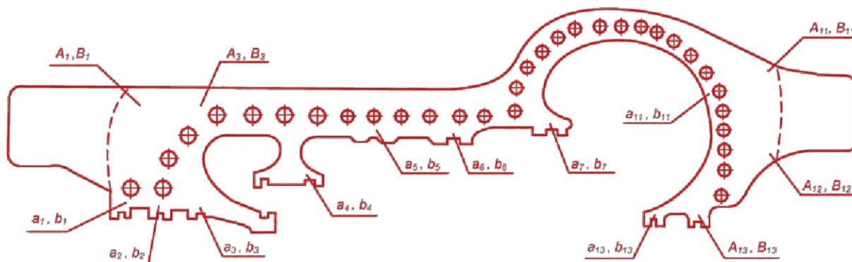
Расчет перемещений деталей проточной части при затяжке корпуса ЦСД-1
