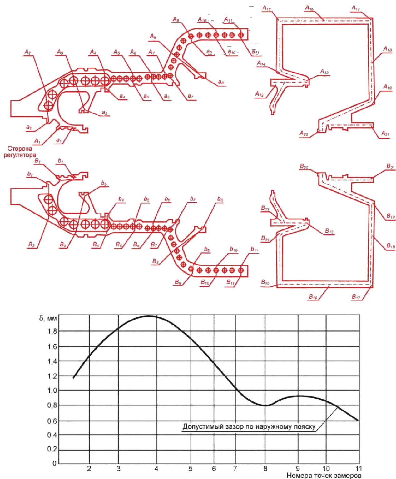
Рисунок Б.8 — Турбина К-300-240 ХТЗ (ЦСД)
