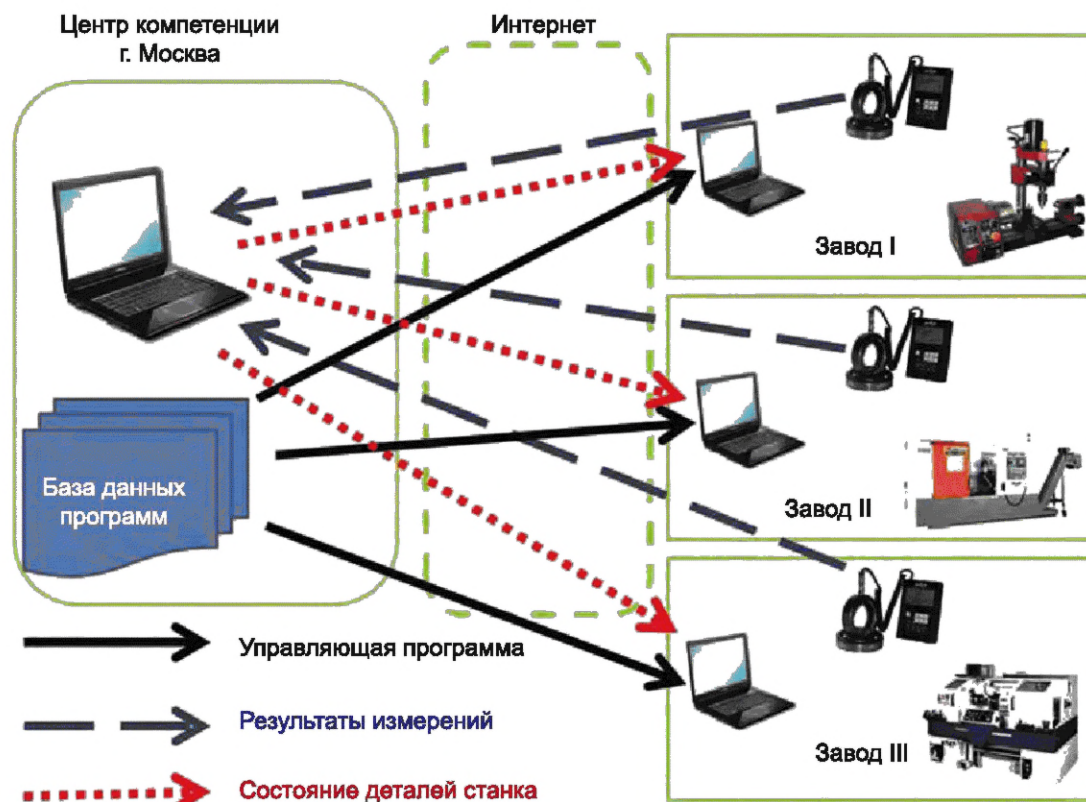
Рисунок Г.3 — Схема удаленной диагностики станков
