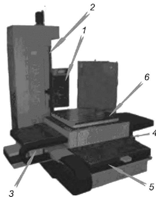
Рисунок Д.9 — Схема расположения точек измерения для вибродиагностики горизонтально-расточного станка модели 2Б622Ф4
