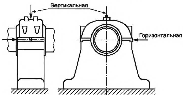
Рисунок В.1 — Точки измерения на опорах подшипника
