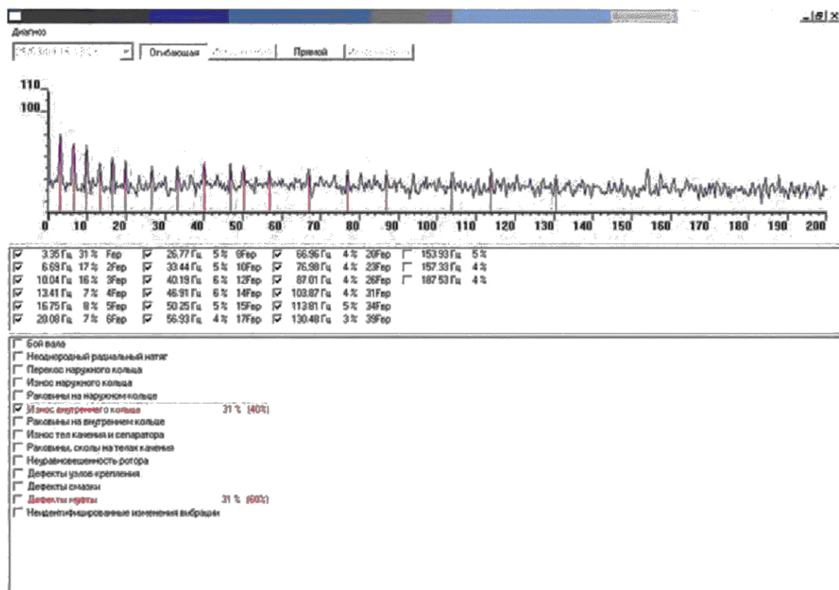
Рисунок Д.10 — График спектра огибающей станка модели 2В622Ф4
