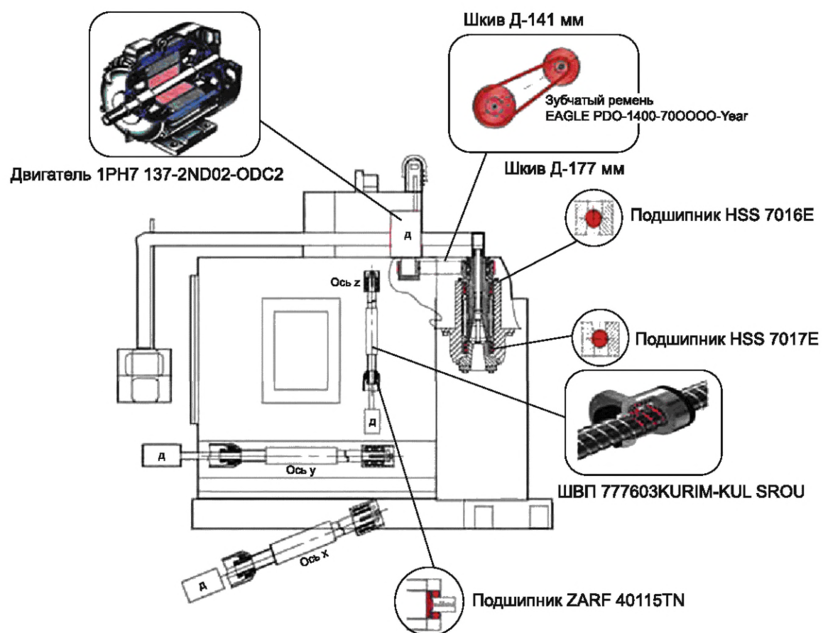
Рисунок Б.3 — Схема состояния деталей станка 1 М512 МФ3 №1
