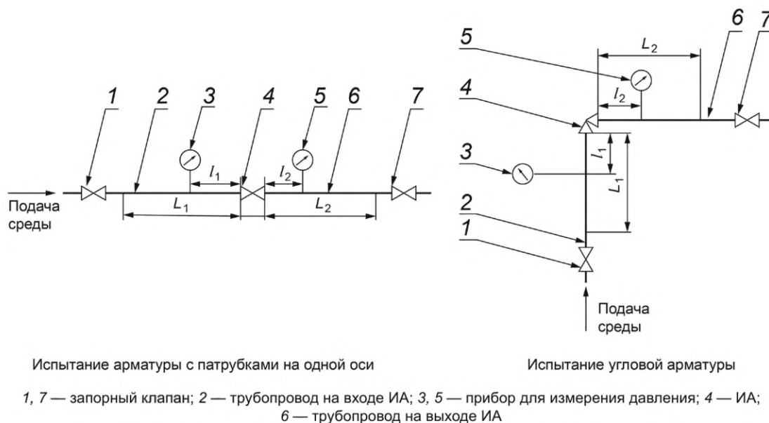
Рисунок 1 — Принципиальная схема испытательного участка гидравлического (пневматического) стенда
