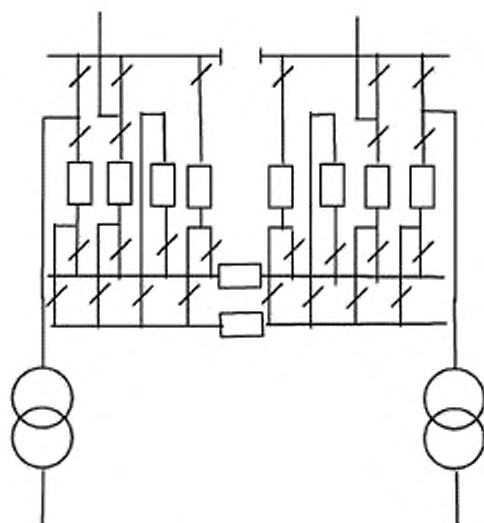
Рисунок А.17 — Схема 14. Две рабочие секционированные выключателями и обходная системы шин с двумя обходными и двумя шинносоединительными выключателями
