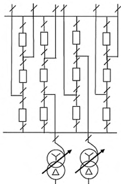
Рисунок А.19 — Схема 17. Полуторная схема
