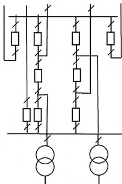
Рисунок А.12 — Схема 9АН. Одна рабочая секционированная система шин с подключением ответственных присоединений через «полупотрону» цепочку
