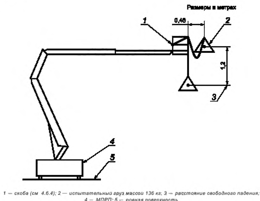
Рисунок 10 — Испытание скоб для крепления устройств предохранения от падения
