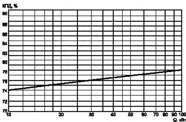
Рисунок 4 — График зависимости КПД котлов для сжигания каменного угля с выходом летучих веществ до 17 % от теплопроизводительности
