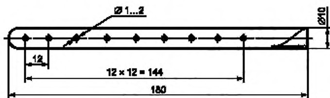
Рисунок 6 — Пробоотборник
