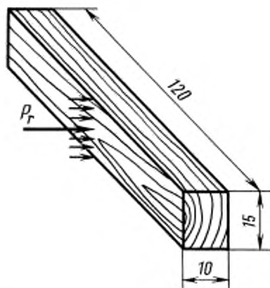
P_r — действие силы удара в радиальном направлении
