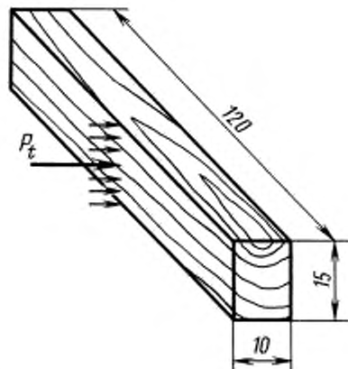
P_t — действие силы удара в тангентальном направлении
