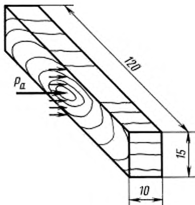
P_a — действие силы удара вдоль волокон (в торце)
