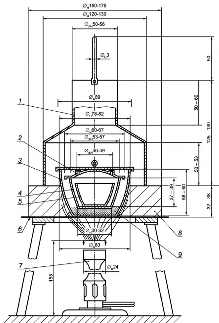
1 — кожух; 2 — горизонтальное отверстие (диаметр примерно 6,5 мм); 3 — тигель из листовой стали (толщина 0,8 мм); 4 — стальной тигель Скидмора вместимостью 65—82 см 3 ; 5 — фарфоровый тигель (вместимостью 29—31 см 3 ); 6 — проволочная подставка из нихрома (калибра № 13 Брауна-Шерпа) или равноценного материала; 7 — горелка Мекера (или равноценная); 8 — теплоизолятор; 9 — сухой песок объемом примерно 25 см 3
