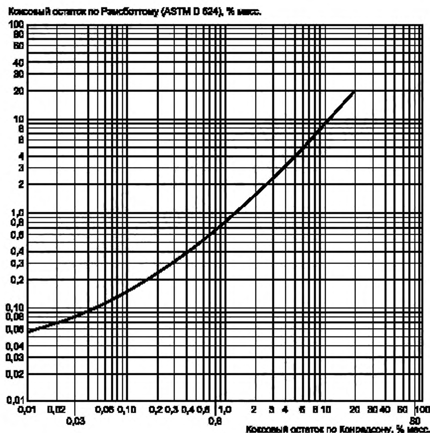
Рисунок X1.1 — Данные корреляции коксового остатка по Конрадсону и Рэмботтону
