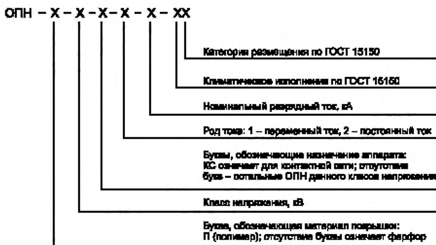
Рисунок 1 — Рекомендуемая структура обозначения ОПН
