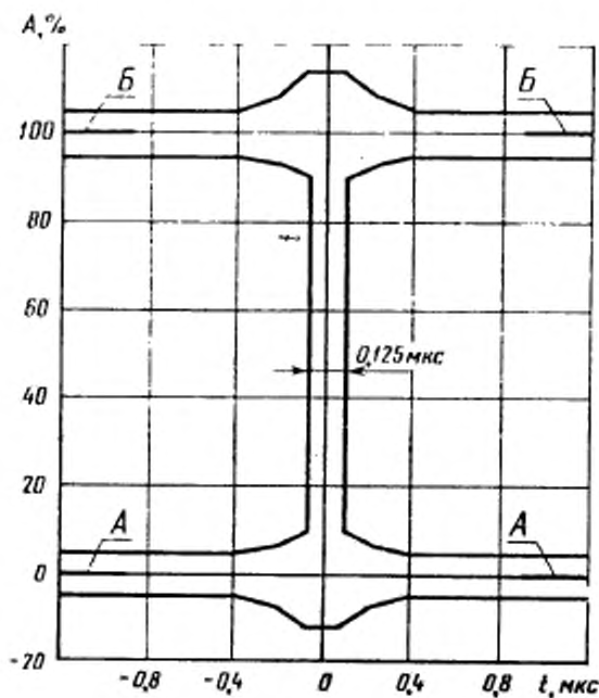
Поле допуска переходной характеристики
