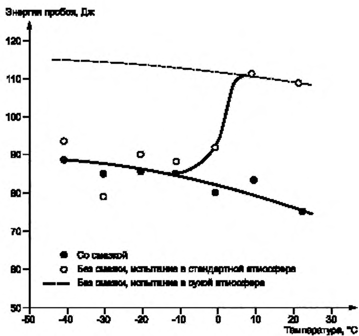
Рисунок В.2 — Зависимость энергии пробова от температуры при использовании смазки и без нее
