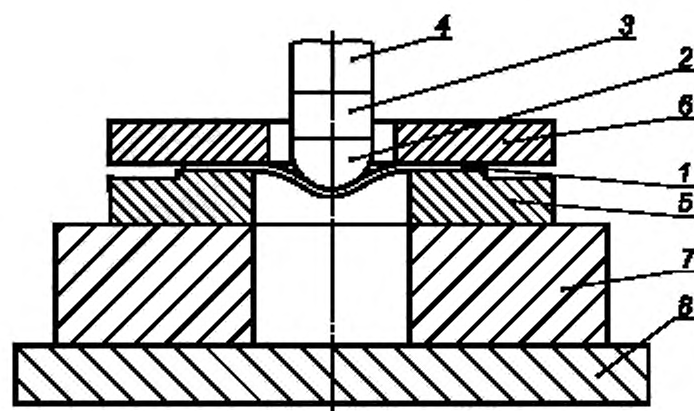
1 — испытуемый образец; 2 — полусферический кончик бойка; 3 — датчик нагрузки (предпочтительное расположение); 4 — стержень; 5 — опора испытуемого образца; 6 — зажимное кольцо (не обязательно); 7 — основание; 8 — акустическая изоляция (не обязательно)
