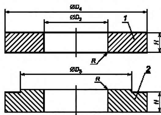
1 — зажимное кольцо (не обязательно), 2 — опора испытуемого образца
