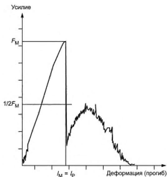
Рисунок А.2 — Схематическое изображение диаграммы «усилие — деформация (прогиб)» для хрупкого или армированного волокном материала
