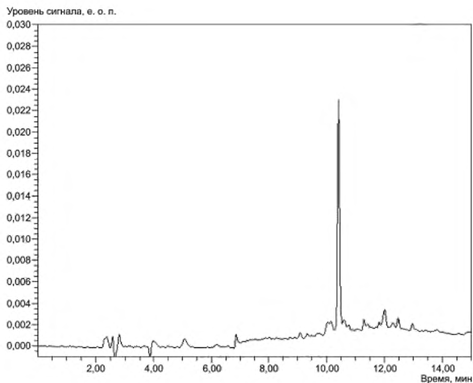
Рисунок Б.2 — Хроматограмма апельсинового сока без СПК
