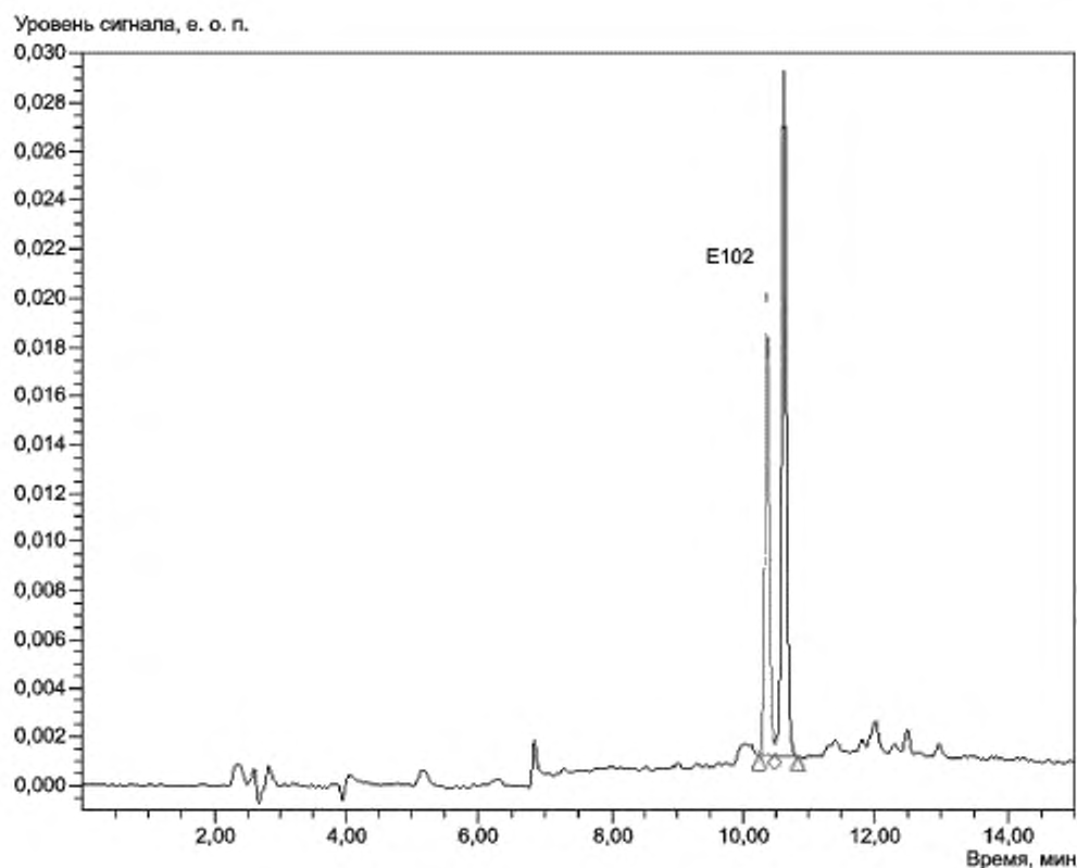
Рисунок Б.3 — Хроматограмма апельсинового сока с добавкой СПК Тартразин (E102), 10 мг/дм 3
