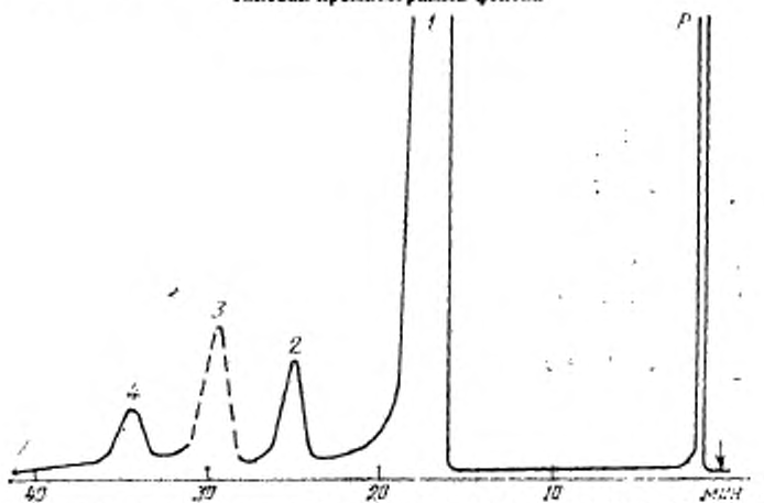
Типовая хроматограмма фенола
