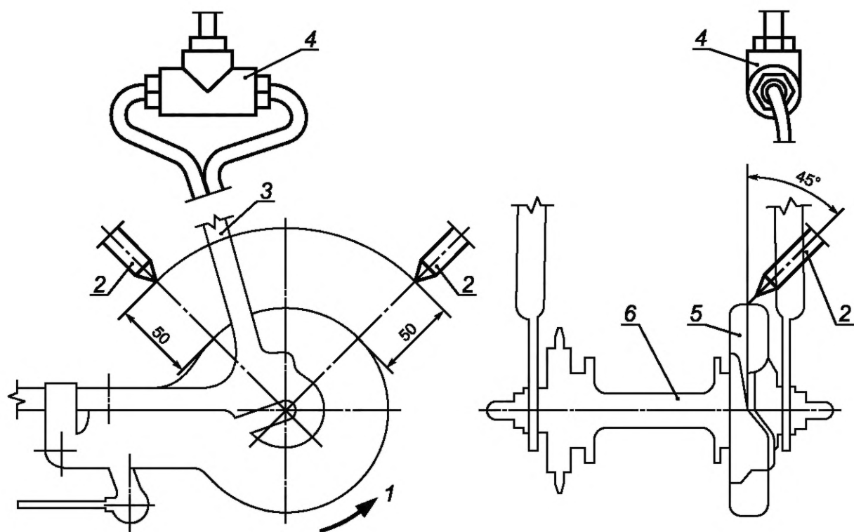
Рисунок 9 — Патрубки для подачи воды для ленточного тормоза
